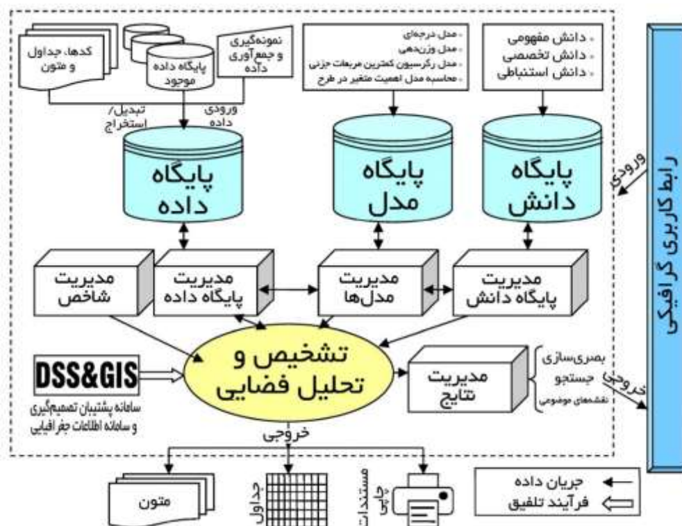
شکل ۶: معماری سامانه پشتیبان تصمیم‌گیری فضایی
